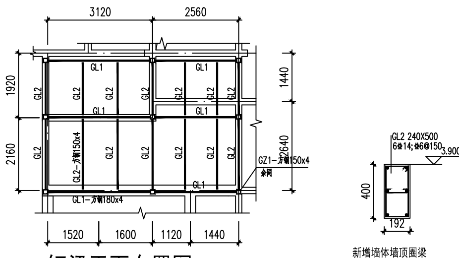
钢梁平面布置图
